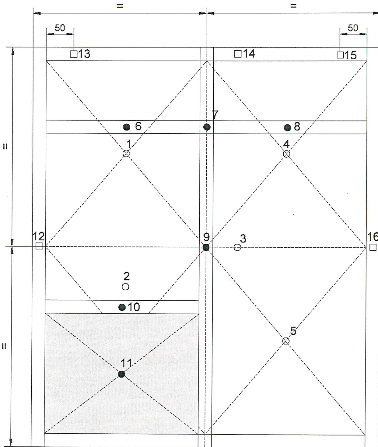
Рис. 1. Схема размещения термопар на образце.
