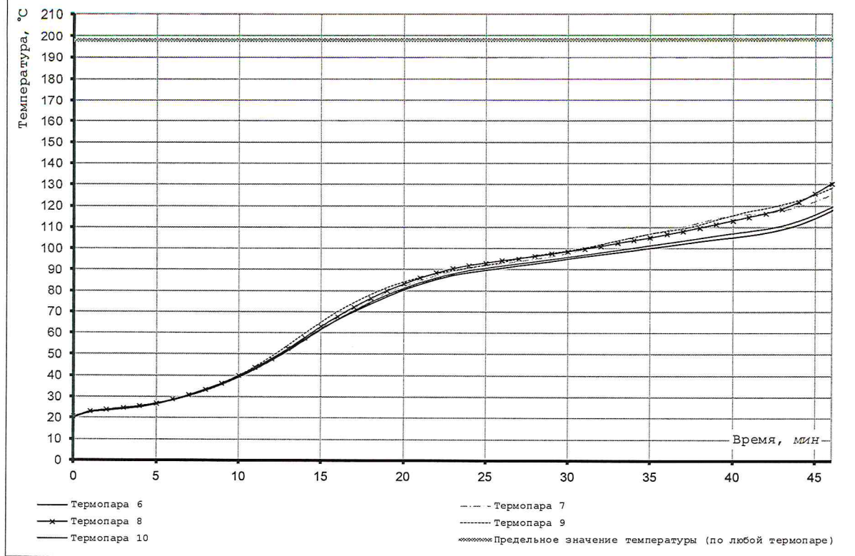
Рис. 10. Образец №2. Измерения температуры на необогреваемой поверхности профилей.
