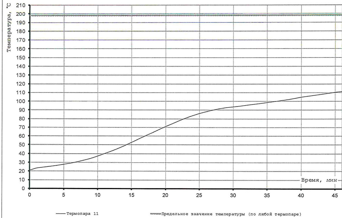
Рис. 6. Образец №1. Измерения температуры на необогреваемой поверхности глухой части.
