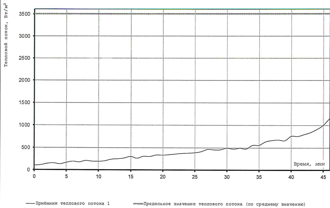
Рис. 8. Образец №1. Измерения плотности потока теплового излучения.
